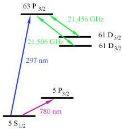
Niveau-Schema ^{85}\text{Rb}
