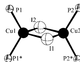
Abbildung 1. Nummerierung und Koordinationsmuster der \text{Cu}_2\text{I}_2 -Rauten und der an Cu koordinierten P-Atome in (\text{CuI})_2\text{P}_8\text{Se}_3 (symmetriegenerierte Atome sind durch einen Stern gekennzeichnet). Die Abstände d(\text{Cu}-\text{I}) sind für I1 etwas länger als für I2. Der Grund dafür sind die größeren Winkel \angle(\text{I}-\text{Cu}-\text{P}) für I2.
