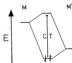
Schema 1. Qualitatives MO-Diagramm einer polaren \text{M–M}' -Bindung mit \text{M}' zu \text{M} CT-Übergang.
