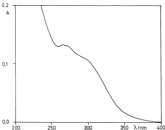
Abb. 1. Absorptionsspektrum von [\text{Ph}_3\text{PAu-Co}(\text{CO})_4] ( 2,4 \times 10^{-5} mol/l) in Hexan gesättigt mit Ar, in einer 1-cm-Küvette.
