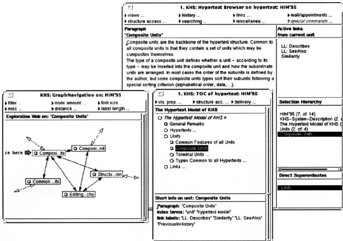
Abbildung 6 Der KHS-Browser in Kooperation mit zwei Übersichtstools, dem in diesem Aufsatz beschriebenen graphischen Browser und einem weiteren, der pseudographische hierarchische strukturelle Beziehungen zwischen Composite Nodes darstellt.
