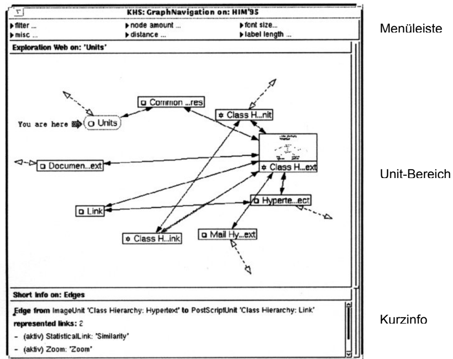
Abbildung 2 Graphische Übersicht ausgehend von der Unit Units . Eine Image-Unit ist ikonisch dargestellt. 4 Verknüpfungen verweisen aus der Übersicht hinaus. Es wird Kurzinformation über die Links präsentiert, die von der Image-Unit Class Hierarchy: Hypertext auf die Unit Class Hierarchy: Link verweisen 2 .
