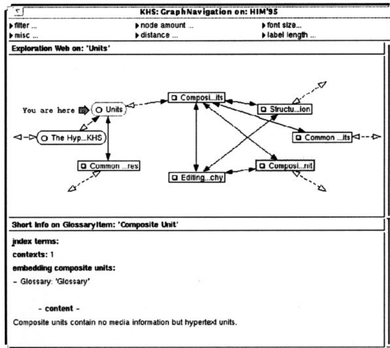
Abbildung 5 Im Vergleich zu Abb. 2 sind hier die Image-Units herausgefiltert, dafür zusätzliche Link-Typen aktiviert. Es wird Kurzinformation zur Glossar-Unit Composite-Unit gegeben. Der Leser hat hier der textuellen Darstellung durch Verschieben des am Fensterrand befindlichen Sliders mehr Platz eingeräumt. Es sind zwei inaktive Kanten sichtbar.
