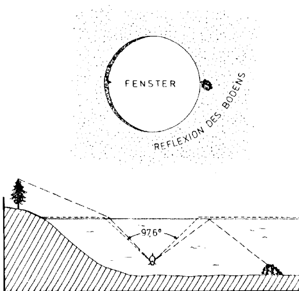
Abb. 6: Der Blick aus dem Wasser. Oben: Das SNELLIUS'sche Fenster in der Wasseroberfläche, durch das Licht von außen hereinfällt. Unten: Innerhalb eines Winkels von 97,6^\circ kann der Fisch die gesamte, über dem Wasser liegende Hemisphäre - zusammengepreßt - sehen. Ausserhalb des Fensters werden die vom Boden reflektierten Objekte gesehen.
