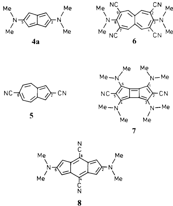
Schema 5. Verringerung der Differenz der Grenzorbitalenergien durch gezieltes Substitutionsmuster (Verbindungen der Kategorie II).
