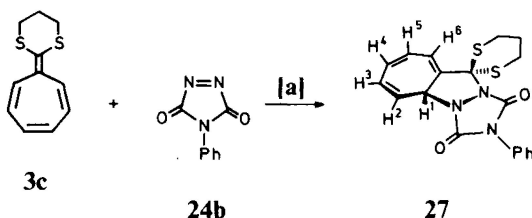
Schema 13. [8 + 2]-Cycloaddition von 8,8-(Trimethylendithio)heptafulven ( 3c ) mit 4-Phenyltriazolindion ( 24b ).
