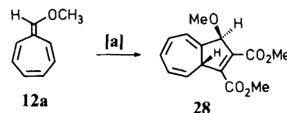
Schema 14. [8 + 2]-Cycloaddition von 8-Methoxyheptafulven ( 12a ) mit Acetylendicarbonsäuredimethylester ( 24c ).
