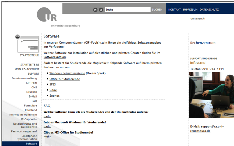
Abbildung 15: Überblick Softwareangebot
