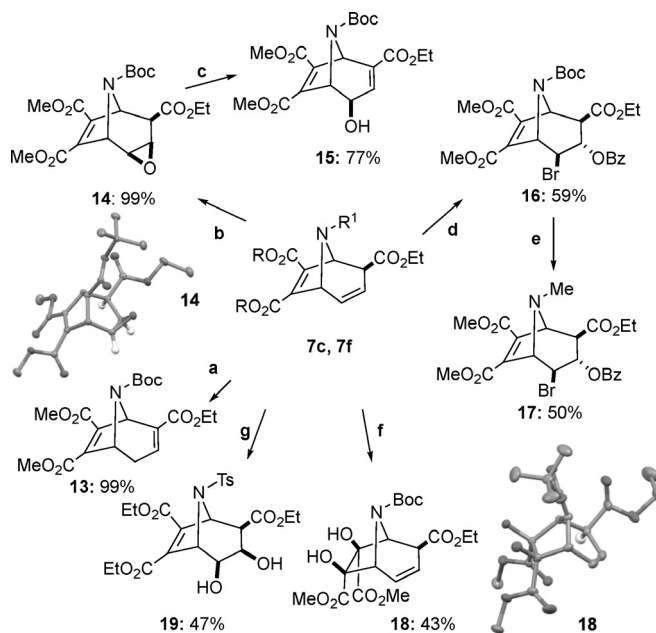
Scheme 6. Derivatierungsreaktionen des 8-Azabicyclo[3.2.1]octan-Gerüsts 7c und 7f . Bedingungen: a) TEA (1.3 Äq.), CH 2 Cl 2 , 2 h, 99%; b) m CPBA (4.0 Äq.), CH 2 Cl 2 , 25 °C, 3 d, 99%; c) Flash Chromatographie, 1% TEA, 77%; d) (i) NBS (2.0 Äq.), Aceton/H 2 O (3:1 v/v), 0 bis 25 °C, 21 h; (ii) BzCl (1.5 Äq.), DMAP (0.5 Äq.), TEA (5.0 Äq.), CH 2 Cl 2 , 25 °C, 8 h, 59%; e) (i) TFA (33 Äq.), CH 2 Cl 2 , 25 °C, 1.5 h, (ii) 37% aq CH 2 O (6.0 Äq.), NaBH 3 CN (3.0 Äq.), MeCN, 25 °C, 1 h, 50%; f) K 2 O 8 ·2H 2 O (0.05 Äq.), NMO (2.0 Äq.), H 2 O, Aceton, 0 °C, 12 h, 43%; g) RuCl 3 ·3H 2 O (6 Mol%), NaIO 4 (1.6 Äq.), MeCN, H 2 O, 0 bis 25 °C, 2 d, 47%.
