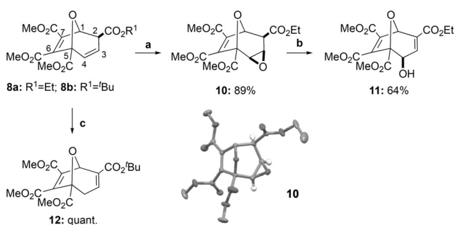
Scheme 5. Derivatierungsreaktionen des 8-Oxabicyclo[3.2.1]octan-Gerüsts 8a,b . Bedingungen: a) m CPBA (3.5 Äq.), CH 2 Cl 2 , 50 °C, 18 h, 89%; b) Flash Chromatographie, 1% Triethylamin (TEA), 64%; c) TEA (1.3 Äq.), CH 2 Cl 2 , 25 °C, 30 min, quant.
