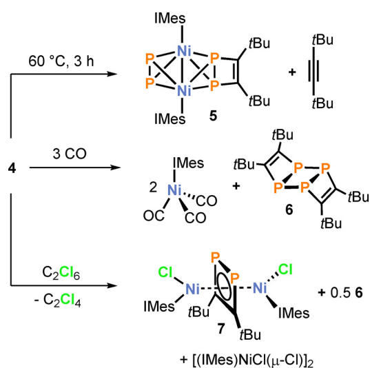
Scheme 2. Reaktivität von 4 beim Erwärmen und bei Zugabe von CO und Hexachlorethan.
