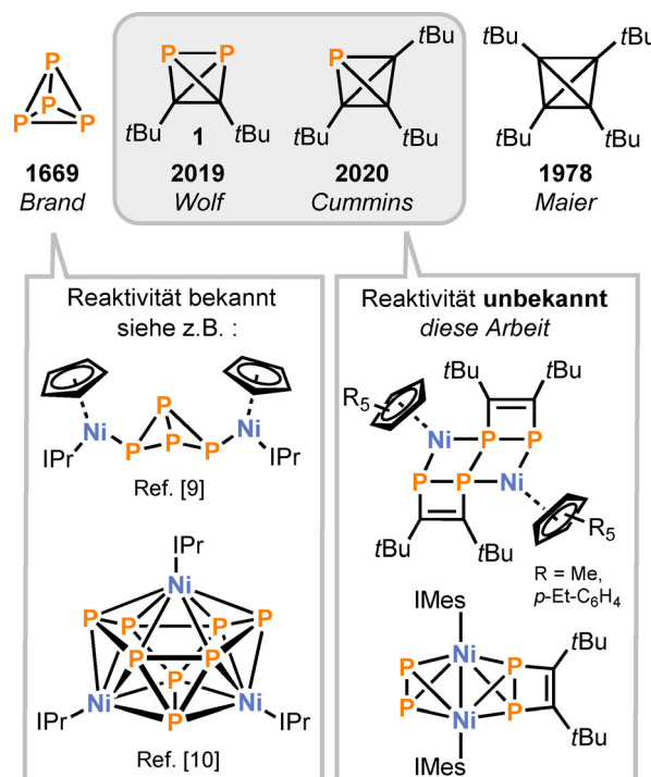
Abbildung 1. (Gemischte) Gruppe-14/15-Tetrahedrane und Reaktivität von P_4 mit NHC-stabilisierten \text{Ni}^{\text{I}} -Metalloradikalen und \text{Ni}^{\text{0}} -Komplexen. [9,10]
