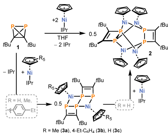
Scheme 1. Reaktionen von [\text{Cp}^{\text{R}}\text{Ni}(\text{IPr})] ( \text{R} = \text{H}; \text{Me}, 4\text{-Et-C}_6\text{H}_4 ) mit (t\text{BuCP})_2 ( 1 ).
