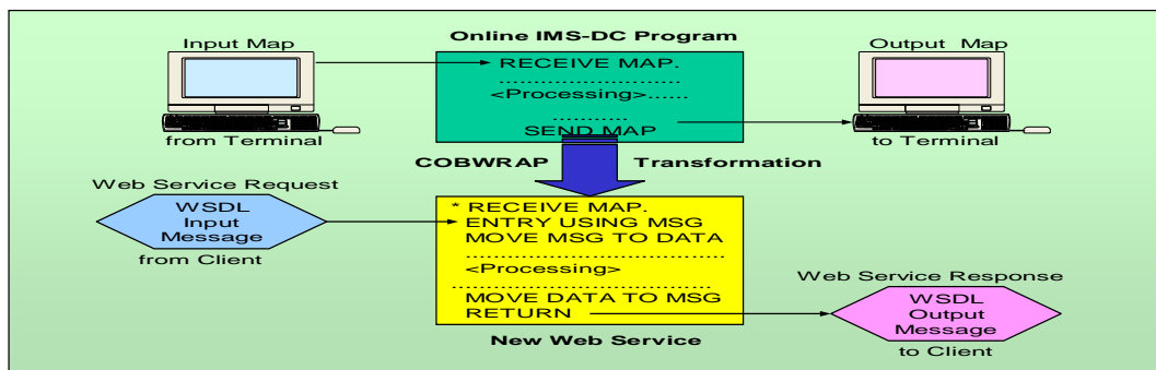
Abbildung 3: Programmkapselung
