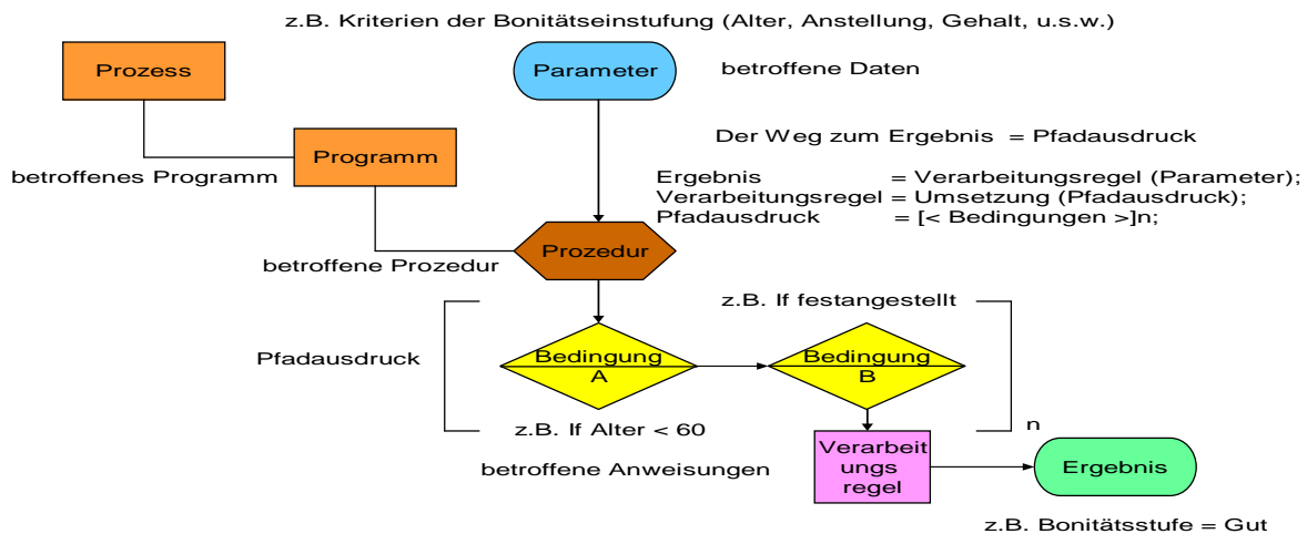
Abbildung 2: Pfadauswahl
