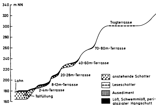
Abb. 1. Schematisches Talquerprofil der Lahn bei Marburg.
